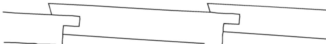
Profilo a scandola per rivestimenti Spessore mm. 25
